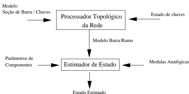
Figura 2: Estimador de estado tradicional
