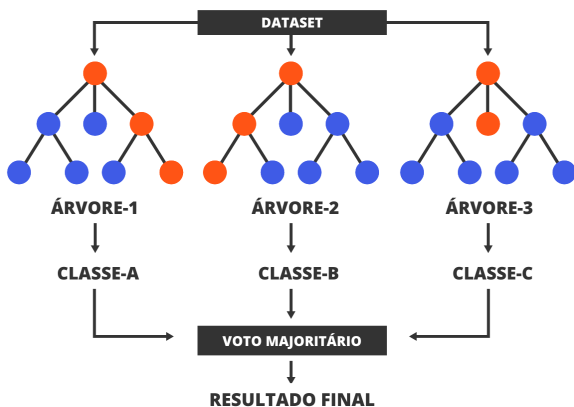
Figura 2. Representação gráfica de uma floresta aleatória
