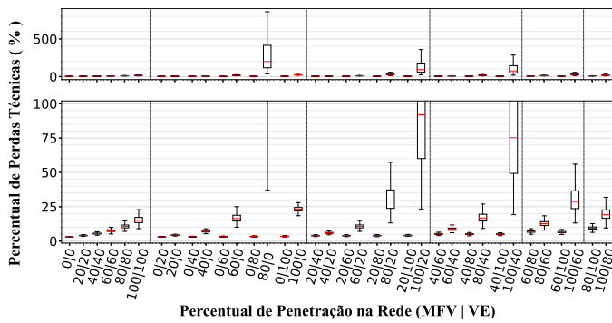
Figura 13. Perdas técnicas para distintos níveis de penetração.
