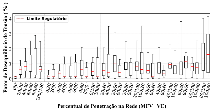
Figura 9. Desequilíbrio de tensão para distintos níveis de penetração.
