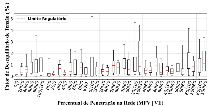
Figura 12. Desequilíbrio de tensão para distintos níveis de penetração e controle Volt-VAR.
