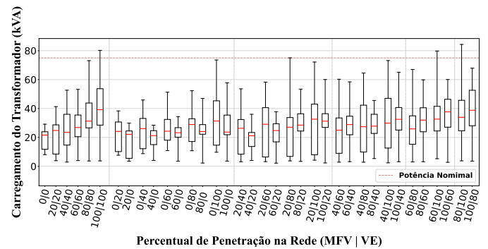
Figura 8. Carregamento do transformador para distintos níveis de penetração.
