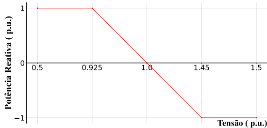
Figura 6. Curva Volt-VAr
