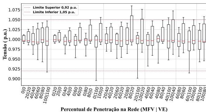
Figura 10. Nível de tensão na RDBT para distintos níveis de penetração de MFV e VE e controle Volt-VAR.
