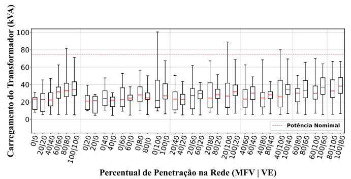
Figura 11. Carregamento do transformador para distintos níveis de penetração e controle Volt-VAR.
