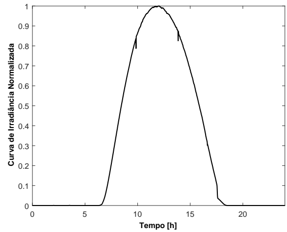
Figura 2. Curva de irradiação solar em dia de céu limpo.
