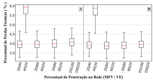
Figura 17. A - Perdas técnicas sem controle VoltVAr, B - Perdas técnicas com controle VoltVAr.
