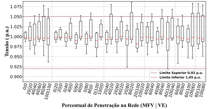
Figura 7. Nível de tensão na RDBT para distintos níveis de penetração de MFV e VE.
