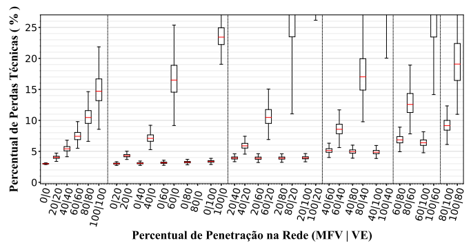
Figura 16. Perdas técnicas para distintos níveis de penetração e controle VoltVAr.
