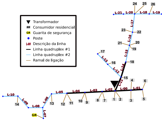
Figura 5. Diagrama unifilar do circuito CA 746.
