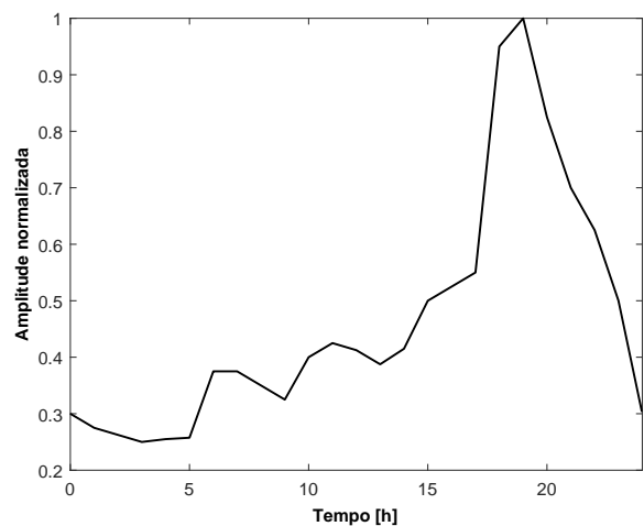
Figura 3. Exemplo de curva de carga residencial.
