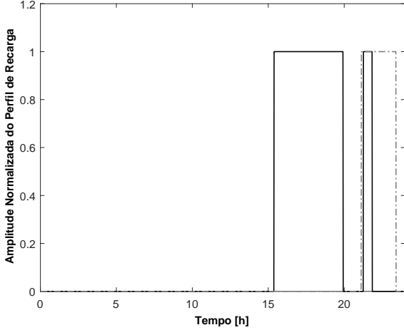
Figura 4. Exemplos de curva de carga de VE para modo lento.
