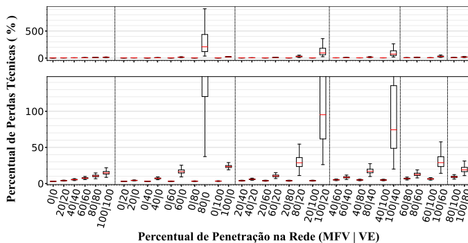
Figura 15. Perdas técnicas para distintos níveis de penetração e controle VoltVAr.
