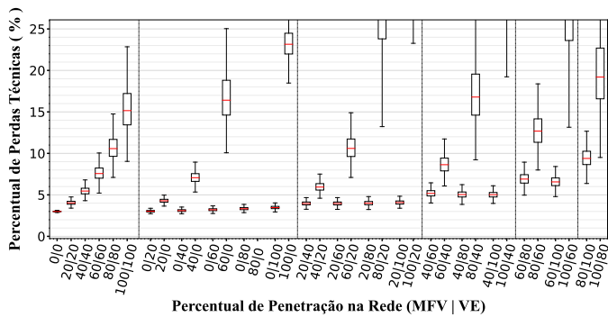
Figura 14. Perdas técnicas para distintos níveis de penetração.
