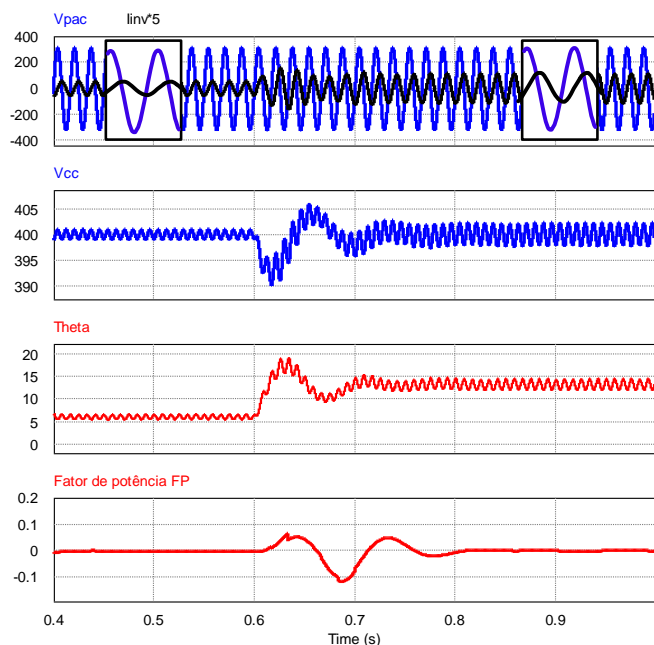
Fig. 12 Resposta dinâmica do sistema ativo quando submetido à degrau de carga.
