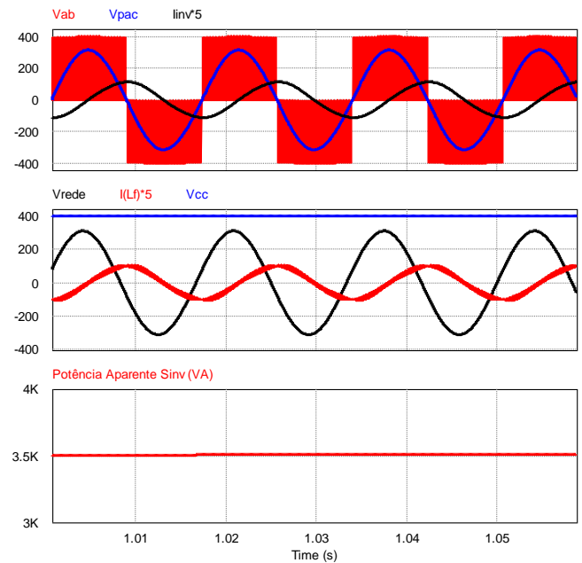
Fig. 11 Tensão V_{ab} no inversor, Tensão no PAC e corrente injetada pelo inversor; Tensão no barramento CC, na rede e Corrente no indutor de filtro do inversor; Potência aparente processada pelo inversor.
