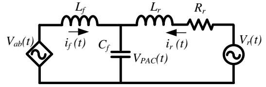
Fig. 6 Circuito equivalente composto pelo filtro LC e rede elétrica.
