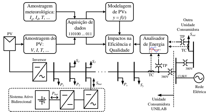
Fig. 1 Esquemático do sistema proposto no projeto estratégico de P&D (Chamada Pública ANEEL nº 01/2016).
