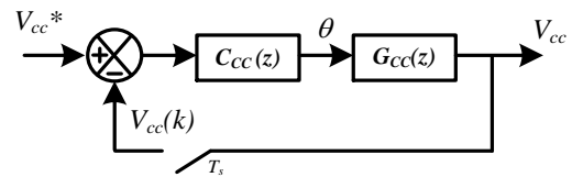
Fig. 7 Malha de controle da tensão no barramento CC.
