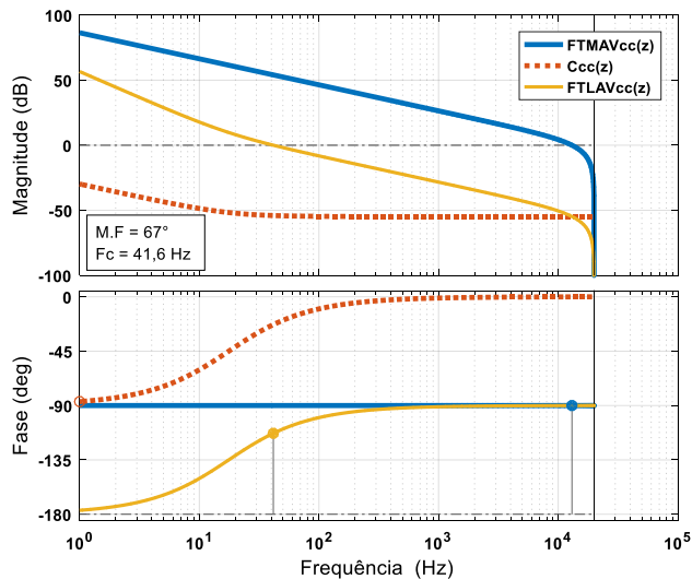
Fig. 10 Diagrama de bode da FTMA não-compensada, FTMA compensada e controlador da malha de tensão no barramento CC.
