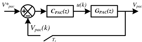
Fig. 5 Malha de controle da tensão do PAC.
