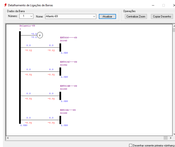
Figura 5. Simulação do Litoral Norte sem carga no ANAREDE.
